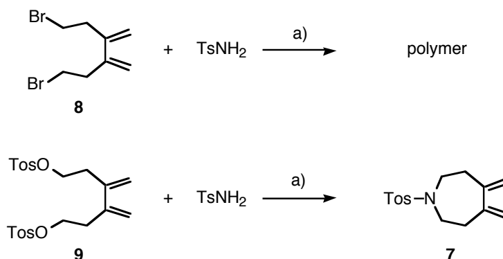
Scheme 2. a) \text{K}_2\text{CO}_3/\text{DMSO} .
