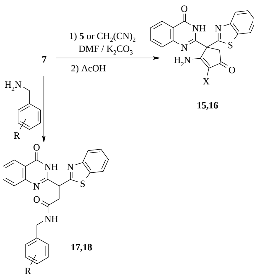
Scheme 3. 15 : \text{X} = 2\text{-benzothiazolyl} , 16 : \text{X} = \text{CN} ; 17 : \text{R} = \text{H} , 18 : \text{R} = 3,4\text{-CH}_2\text{O}_2
