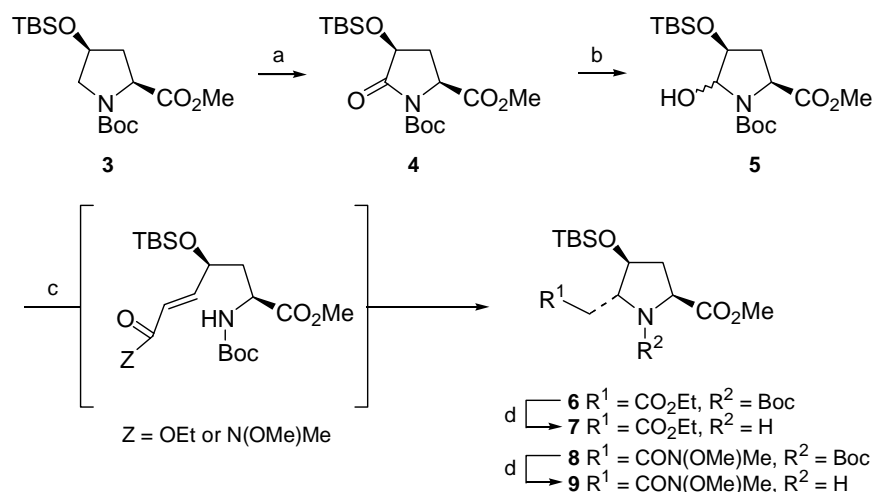
Scheme 1. Reagents and conditions: (a) RuO 2 (cat), NaIO 4 , AcOEt/H 2 O, rt (86%); (b) LiEt 3 BH, THF, -78°C; (c) (EtO) 2 P(O)CH 2 CO 2 Et or (EtO) 2 P(O)CH 2 CON(OMe)Me, NaH, THF, rt ( 6 : 62% from 4 , 8 : 83% from 4 ); (d) TFA, CH 2 Cl 2 , 0°C ~ rt ( 7 : 53%, 9 : 56%).
