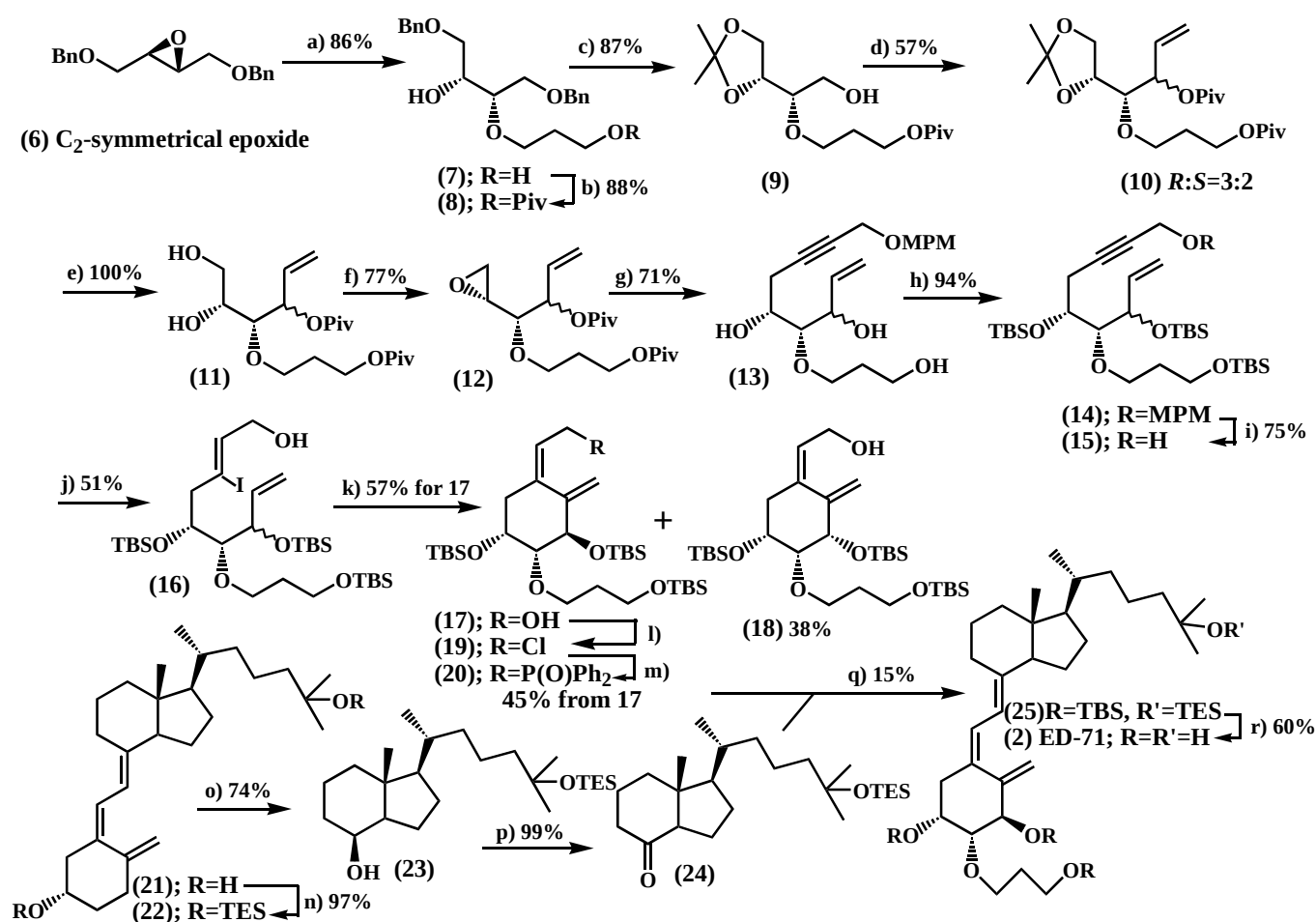
Scheme 2. First convergent synthesis of ED-71 by the Lythgoe coupling reaction. Reagents and conditions: a) HO(CH 2 ) 3 OH/ t -BuOK, 120°C. b) t -BuCOCl/pyridine/CH 2 Cl 2 , rt. c) 1) H 2 /Pd(OH) 2 /MeOH, rt. 2) Me 2 C(OMe) 2 /TsOH/acetone, rt. d) 1) DMSO/(COCl) 2 /CH 2 Cl 2 , -60°C. 2) CH 2 =CHMgBr/THF, -60°C. 3) t -BuCOCl/Et 3 N/DMAP/CH 2 Cl 2 , rt. e) 1M HCl/MeOH, rt. f) Ph 3 P/DEAD/benzene, reflux. g) 1) LiC≡CCH 2 OMPM/BF 3 ·OEt 2 /THF, -60°C~-10°C. 2) 10M NaOH/MeOH, reflux. h) TBSOTf/Et 3 N/CH 2 Cl 2 , 0°C, i) DDQ/CH 2 Cl 2 , rt. j) Red-Al/Et 2 O/toluene, 0°C~rt, then I 2 /AcOEt, -78°C. k) PdCl 2 (PPh 3 ) 2 /Et 3 N/MeCN, reflux. l) NCS/Me 2 S/CH 2 Cl 2 , -20°C. m) 1) LiPPh 2 /THF, -78°C. 2) H 2 O 2 , 0°C. n) TESOTf/Et 3 N/CH 2 Cl 2 , 0°C. o) O 3 /CH 2 Cl 2 /MeOH, -78°C then NaBH 4 /MeOH, -78°C. p) NMO/TPAP/4Ams/CH 2 Cl 2 , rt. q) n -Buli/THF, -78°C. r) TBAF/THF.
