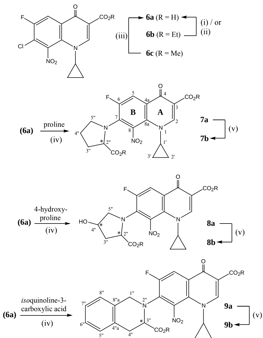
Scheme 1. (i) 4 N HCl / \Delta , 24 h ; (ii) 50 % H 2 SO 4 / \Delta , 2 h (iii) AcOH + H 2 O + H 2 SO 4 (8 : 7 : 1, v/v/v) / \Delta , 2 h (iv) NaHCO 3 , 50 % aq. EtOH / \Delta , then 3 N HCl (v) CH 2 N 2 in Et 2 O / 5-10 °C
