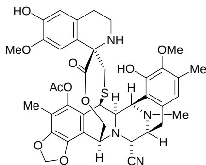
ecteinascidin 770 ( 16 )
