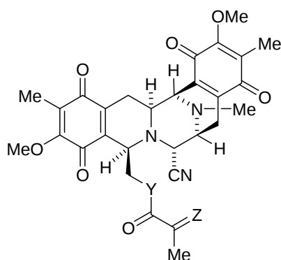
saframycin A ( 14 )
