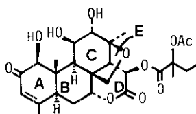
(+)-quassimarin (1)
