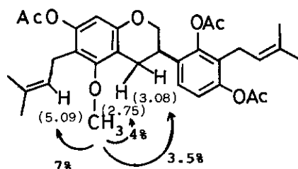
Fig. 4 NOE values for 1a
