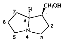
1 Isoretronecanol
