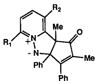
1a; R_1=R_2=H 1b; R_1=H, R_2=Me 1c; R_1=R_2=Me
