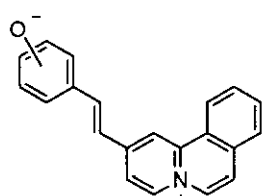
1a: ortho -O - 1b: para -O -
