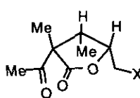
3α X : I 4α X : H 5α X : SPh
