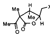
3β X : I 4β X : H 5β X : SPh
