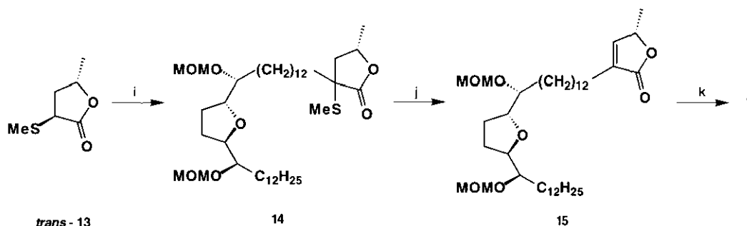
Scheme 4. i) NaHMDS, THF, then 12 , HMPA, 86%. j) m -CPBA, CH 2 Cl 2 . k) tol. , CaCO 3 , Δ, 97%. l) BF 3 ·Et 2 O, SMe 2 , 90%
