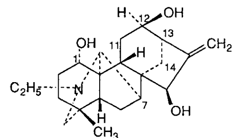
9 12- epi -Napelline
