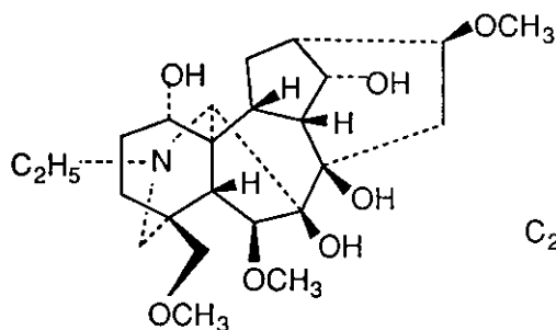
1 Delcosine
