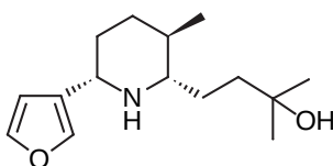
2 (-)-Nupharamine
