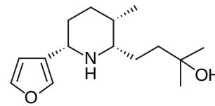
4 (+)-3-Epinupharamine
