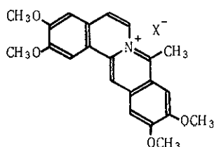
72a X=Cl
