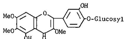
Chrysosplenoside D
