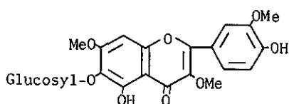
Chrysosplenoside C
