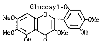
Chrysosplenoside A
