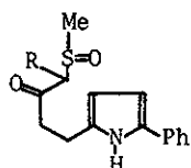
1, R=H 2, R=CONHPh
