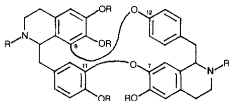
Group 8 * , 11 † -7 † , 12 *
