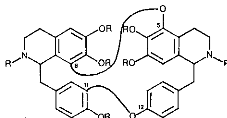
Group 8 * , 11 † -5 * , 12 †
