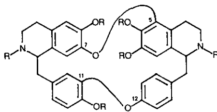
Group 7^*, 11^+ - 5^*, 12^+
