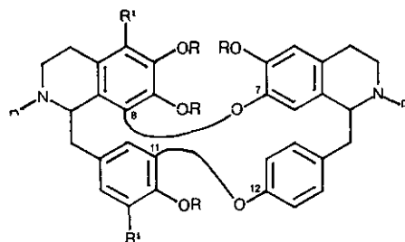
Group 8 * , 11 † -7 * , 12 †
