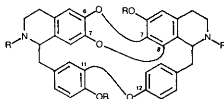
Group 6^*, 7^+, 11^+ - 7^*, 8^+, 12^+
