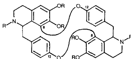
Group 8 * , 12 † -8 † , 12 *
