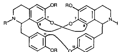
Group 7^*, 8^+, 11^+ - 8^*, 7^+, 12^+
