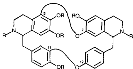
Group 5^*, 11^+ - 7^*, 12^+
