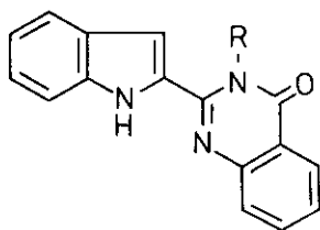
2 a R=H b R=NH 2
