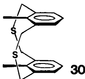
30 syn -isomer; \delta_{\text{CH}_3} = 2.54
