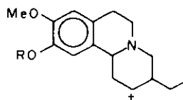
g m/z 302 (R=Ac) g m/z 260 (R=H)
