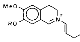
c m/z 274 (R=Ac) h m/z 232 (R=H)
