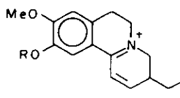
b m/z 300 (R=Ac) d m/z 258 (R=H)
