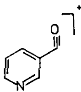
(d) m/z 106
