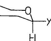
(14) Y : \text{NH}_2
