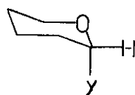
(15) Y : \text{NH}_2
