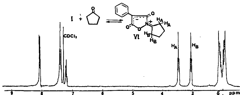
Fig. 4. Hnmr of VI
