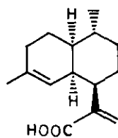
13 : 4,5-ene
