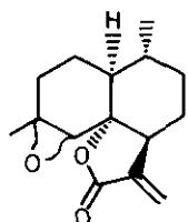
3 : \alpha -epoxy
