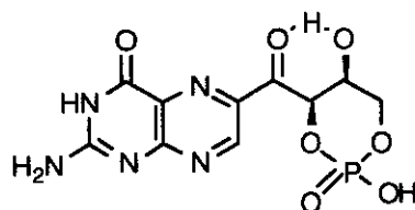
7b : Cis
