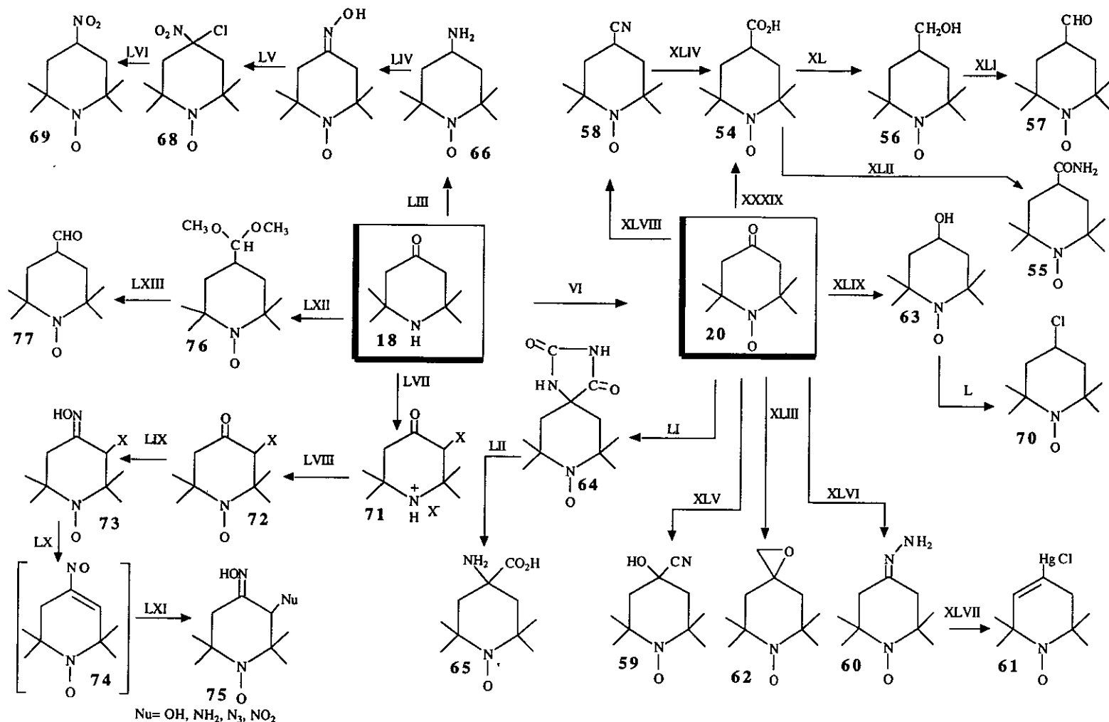
Scheme 4b. XXXIX) 1) TosCH 2 NC, 2) Ba(OH) 2 /H 2 O/100°C 185; XL) Sodium bis(2-methoxyethoxy)aluminium hydride/toluene 176; XLI) MnO 2 /CCl 4 176; XLII) CH 2 N 2 /NH 3 /CH 3 OH 180, 186; XLIII) CTsCH 2 NC/C 4 H 9 OK 185; XLIV) Ba(OH) 2 /NaOH/H 2 O 185; XLV) HCN 189; XLVI) 1) NH 2 NH 2 , 2) K 3 Fe(CN) 6 161, 190; XLVII) Hg(OAc) 2 /CaCl 2 /H 2 O 191; LVIII) (CH 3 ) 3 S + I - /NaH 187; XLIX) LiAlH 4 ; L) SOCl 2 183; LI) KCN/H 2 O/(NH 4 ) 2 CO 3 182; LII) Ba(OH) 2 /100°C 182; LIII) NH 4 OAc/NaBH 3 CN/CH 3 OH 192, 193; LIV) 1) Ac 2 O, 2) H 2 O 2 /Na 2 WO 4 , 3) NaOH/100°C, 15 h 192-195; LV) NaOCl 196-197; LVI) H 2 196-197; LVII) SOCl 2 or Br 2 198; LVIII) 30% H 2 O 2 /Na 2 WO 4 /H 2 O 198; LIX) NH 3 199; LX and LXI) NuH 199; LXII) 1) MCPBA 2) (C 6 H 5 ) 3 P=CH-OCH 3 3) CH 3 OH 200; LXIII) 1) H 2 /Pt, 2) H 2 SO 4 3) (KO 3 ) 2 NO 200.
