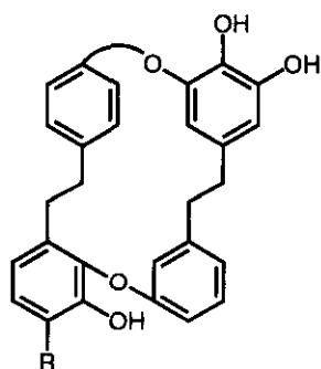
(356) R=H
