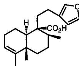
(190)
