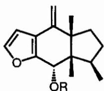
(157) \text{R}=\text{H} (158) \text{R}=\text{Me}
