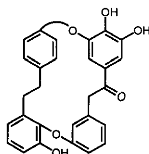
(362)
