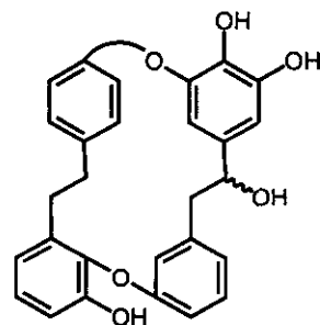
(359)
