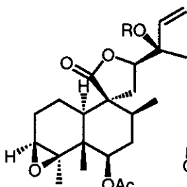
(221) R=Ac (222) R=H
