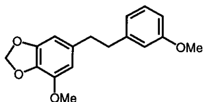
(317)
