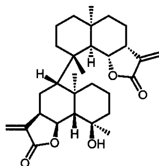
(107)
