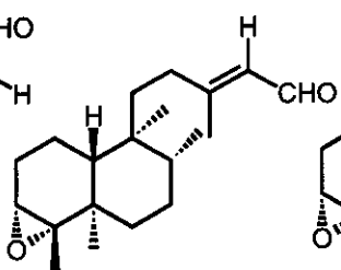
(192)
