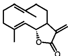
(124)
