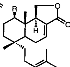
(282) R=H
