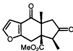
(178)
