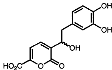
(418)
