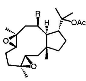
(224) R=OAc (225) R=H
