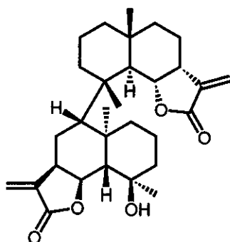
(106)
