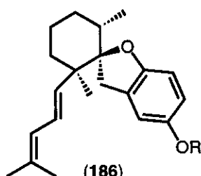
(186)
