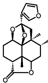
(197)
