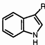
(435) R=CH_2CO_2H (436) R=Me
