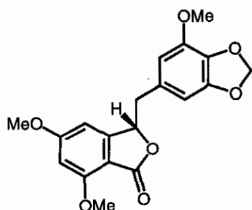
(423)
