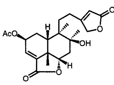
(200)
