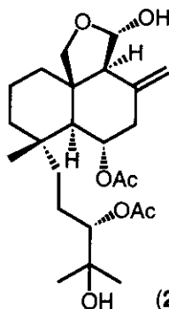
(283) R=OH
