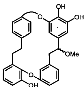
(360)
