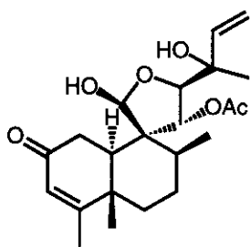
(218)
