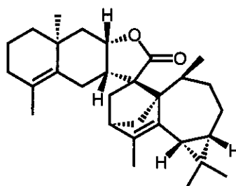
(121)
