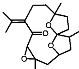
(189)
