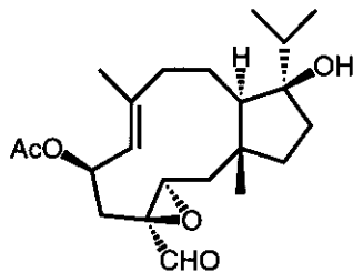
(227)
