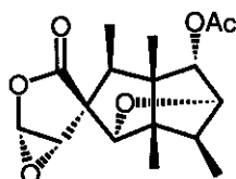
(167)
