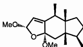
(159)
