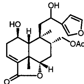
(201)
