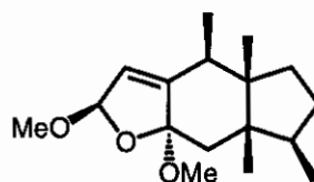
(160)
