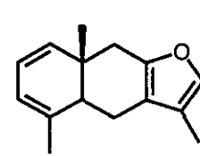
(69)
