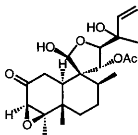
(217)
