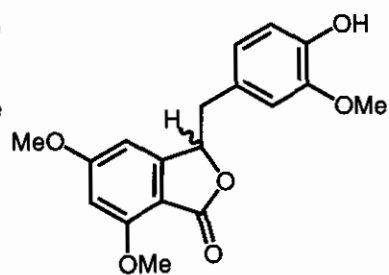
(422)
