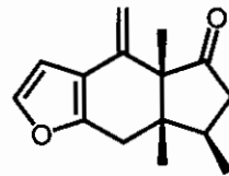
(152)
