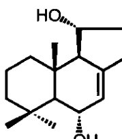
(56)
