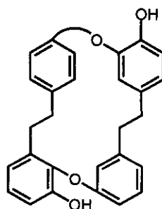
(358)
