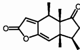
(151)
