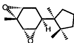
(51)
