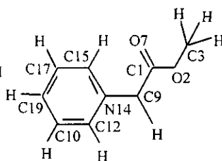
Scheme 17 : Ylide ( G ).
