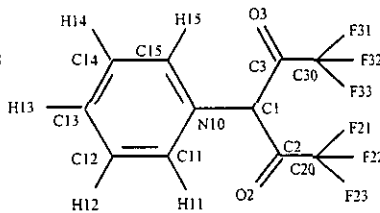
Scheme 10 : Ylide ( D ).
