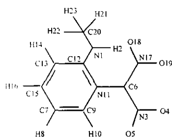
Scheme 9 : Ylide ( C ).
