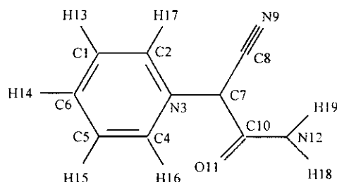
Scheme 8 : Ylide ( B ).
