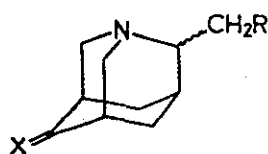
5 X=O R=H 6 X=H 2 R=OH 7 X=O R=OH
