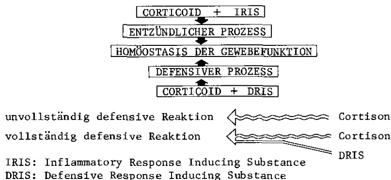
Abb. 6. Schematische Darstellung der Nagais Arbeitshypothese über chemischen Prozesse bei einer Entzündung. (1969)
