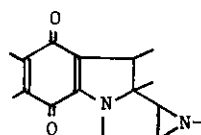
mitosane type
