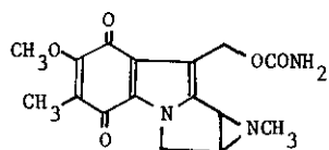
Aziridinomitosene (1)
