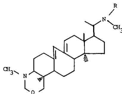
Moenjodaramine (3): R=CH 3
