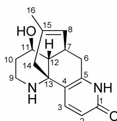
carinatumin B ( 35 )
