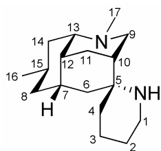
nankakurine A ( 42 )
