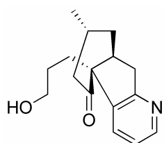
lycoplade A ( 24 ) 44 \text{C}_{16}\text{H}_{21}\text{NO}_2
