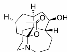
lycoplade D ( 27 ) 45 \text{C}_{16}\text{H}_{23}\text{NO}_3
