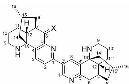
complanadine A : \text{X}=\text{H}_2 complanadine B ( 49 ) : \text{X}=\text{O}
