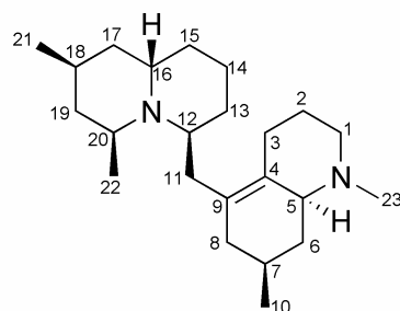
senepodine A
