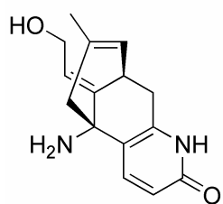
carinatumin A ( 34 ) 49 C 15 H 18 N 2 O 2
