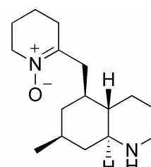
carinatumin C ( 36 ) 49 C 16 H 28 N 2 O
