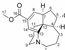
lycopladiene B ( 25 )
