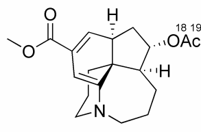
lycopladiene C ( 26 )
