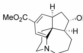
lycoplade B ( 25 ) 45 \text{C}_{17}\text{H}_{23}\text{NO}_3
