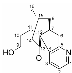
lycopladiene A ( 24 )
