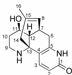
carinatumin B ( 35 )
