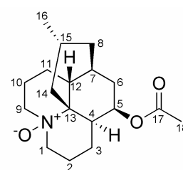
lycopladiene E ( 28 )
