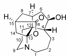
lycopladiene D ( 27 )
