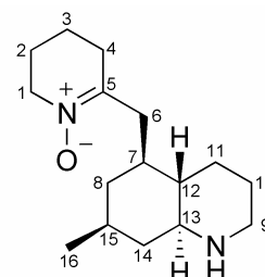
carinatumin C ( 36 )
