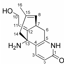
carinatumin A ( 34 )
