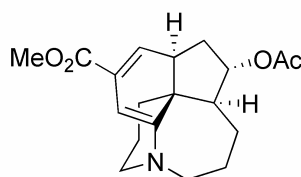
lycoplade C ( 26 ) 45 \text{C}_{19}\text{H}_{25}\text{NO}_4
