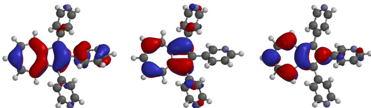
HOMO-1
