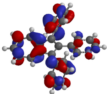
LUMO+2
