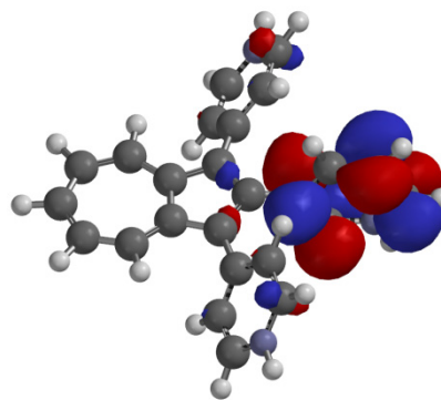
LUMO+4
