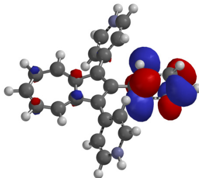
LUMO+3
