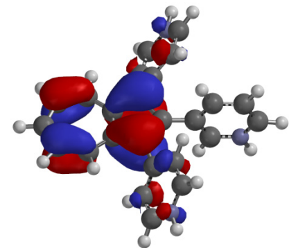
LUMO+2
