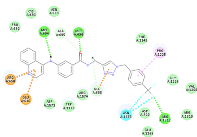
(D) compound F (trifluoromethylphenyl group)
