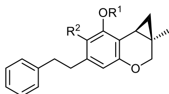
radulanin I ( 31 ) R 1 =R 2 =H
