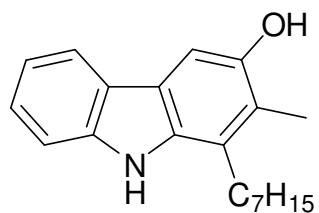
1: Carazostatin
