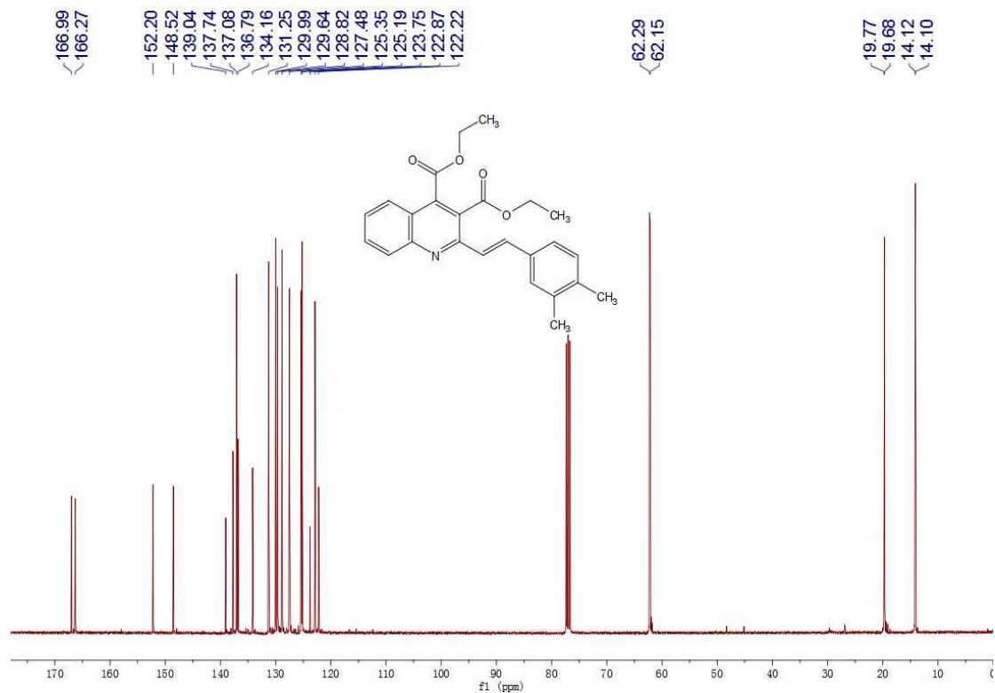
Fig. S10 13 C NMR spectrum of 3e
