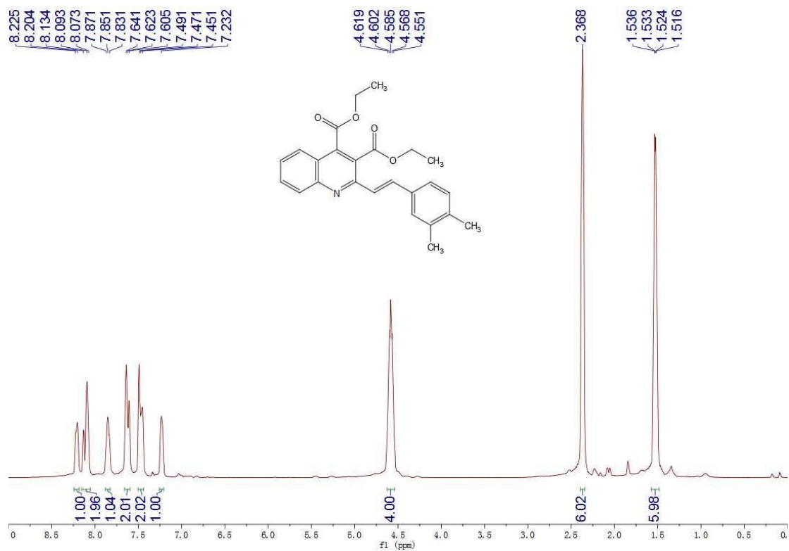
Fig. S9 1 H NMR spectrum of 3e
