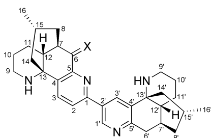
complanadine A : X=H 2 complanadine B ( 49 ) : X=O
