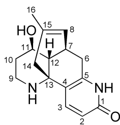
carinatumin B ( 35 )
