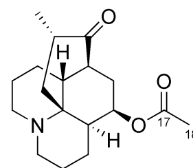
obscurumine B ( 7 )
