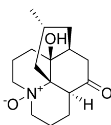
obscurumine A ( 6 )
