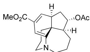
lycopladine C ( 26 ) 45 C 19 H 25 NO 4
