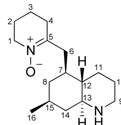
carinatumin C ( 36 )
