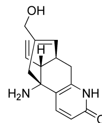
lycoparin C ( 33 ) 48 C 15 H 18 N 2 O 2
