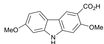
clauszoline-J ( 95 )
