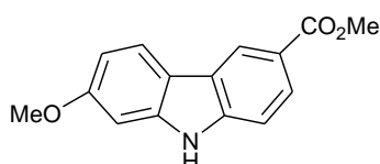
clauszoline-L ( 97 )
