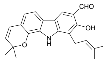
clauszoline-A ( 86 )
