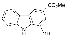
clauszoline-I ( 94 )
