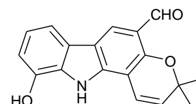
clauszoline-G ( 92 )
