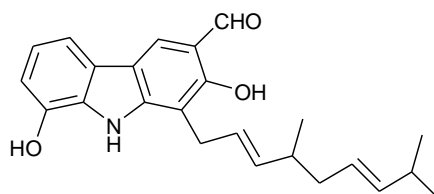
clauszoline-F ( 91 )
