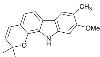
clauszoline-H ( 93 )
