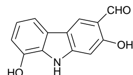
clauszoline-M ( 98 )
