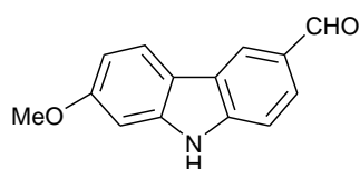
clauszoline-K ( 96 )
