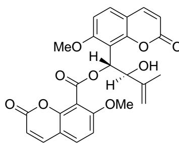
cladimarin B (53)
