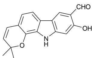
clauszoline-B ( 87 )
