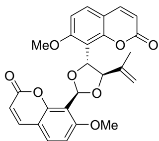
cladimarin A (52)
