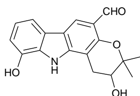
clauszoline-E ( 90 )
