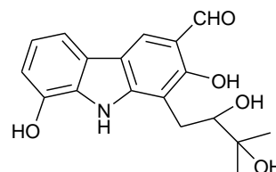
clauszoline-D ( 89 )
