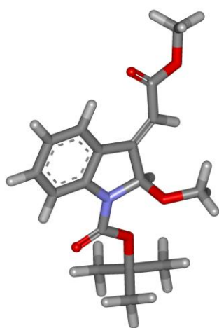
s-trans-(E)-12
