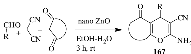
Scheme 135
