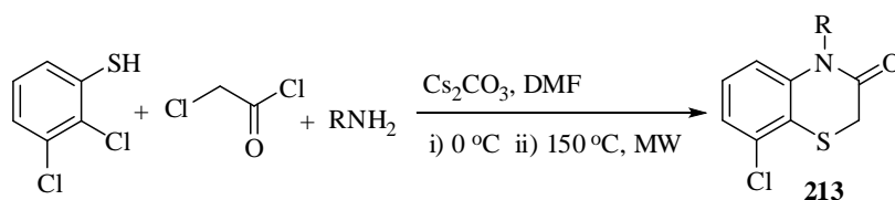
Scheme 170
