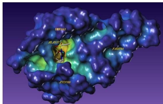
Figure 5. Active pocket of ALS occupied by Safener 4k
