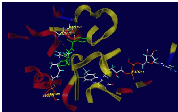
Figure 4. Safener 4k in the ALS active site
